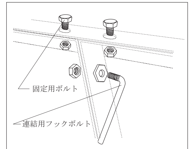
連結用フックボルト 組立詳細図
