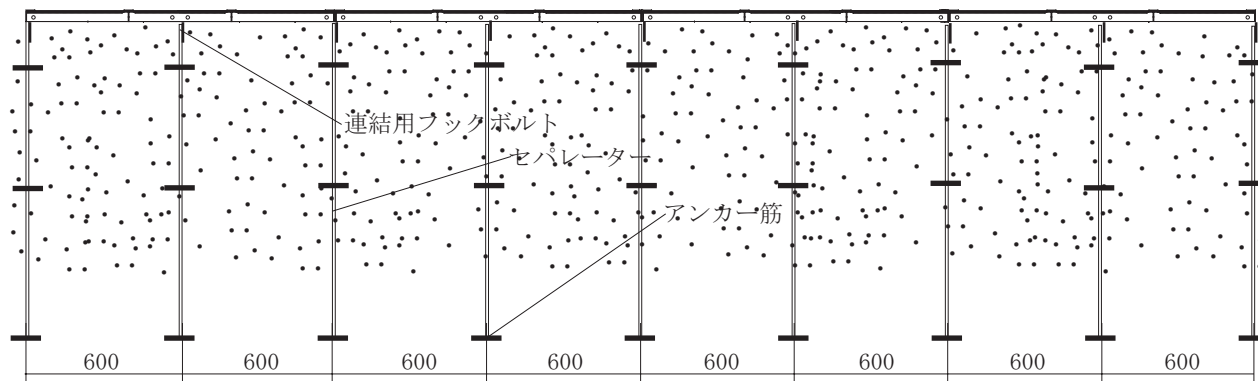
B~B' 断面図
