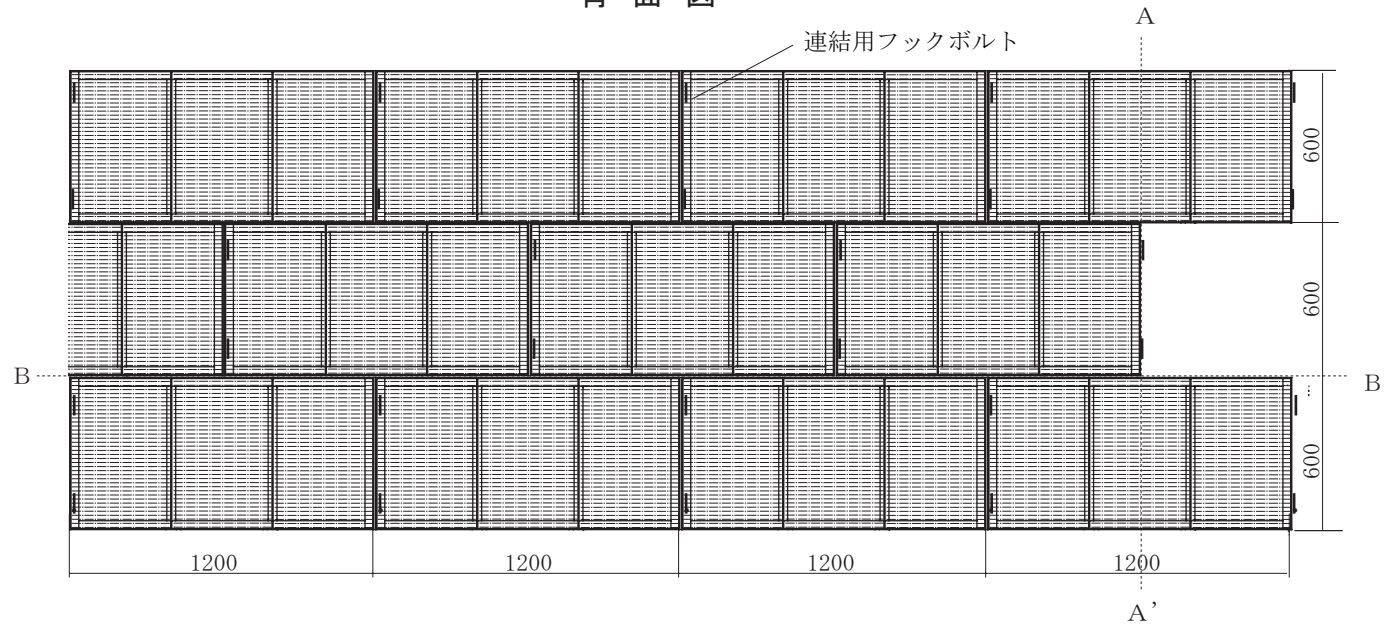
背面図
