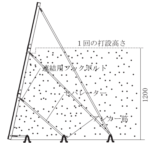
A~A' 断面図
